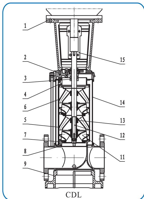
截面图 CDL,CDLF120,150,200
