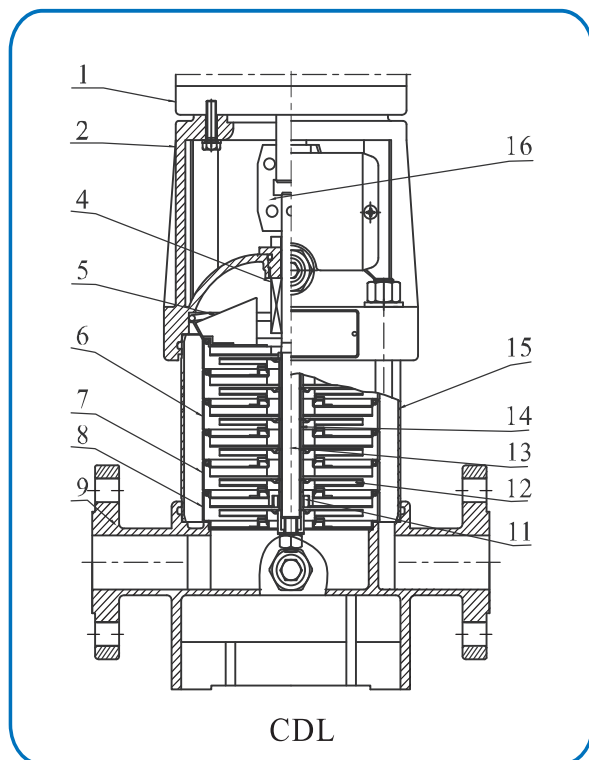
截面图 CDL,CDLF1,2,3,4,5
