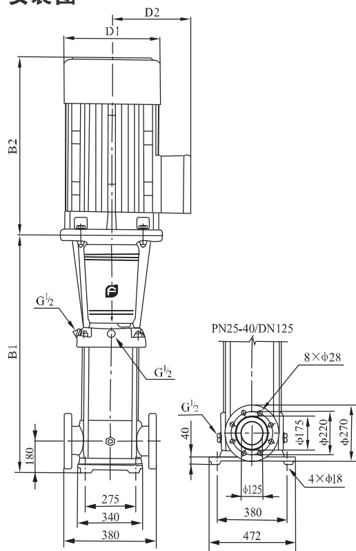
安装图
