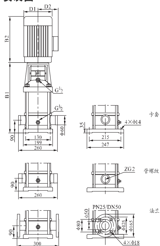
安装图
