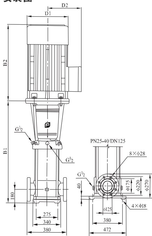
安装图
