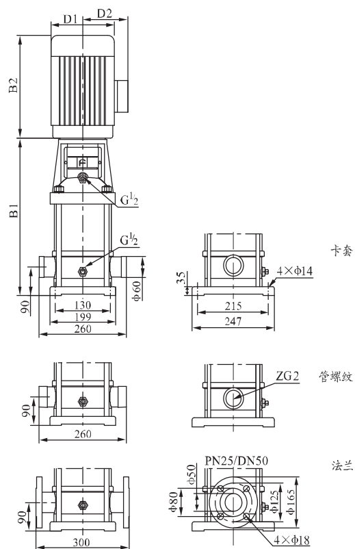
安装图
