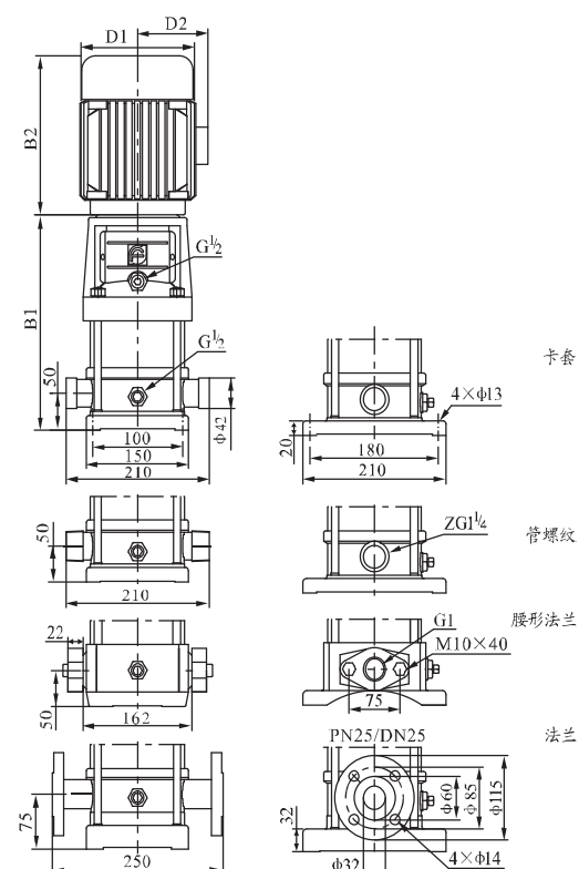
安装图
