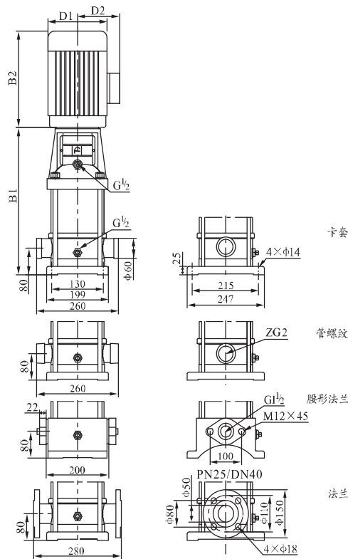
安装图
