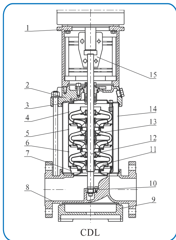
截面图 CDL,CDLF32,42,65,85
