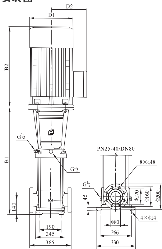
安装图
